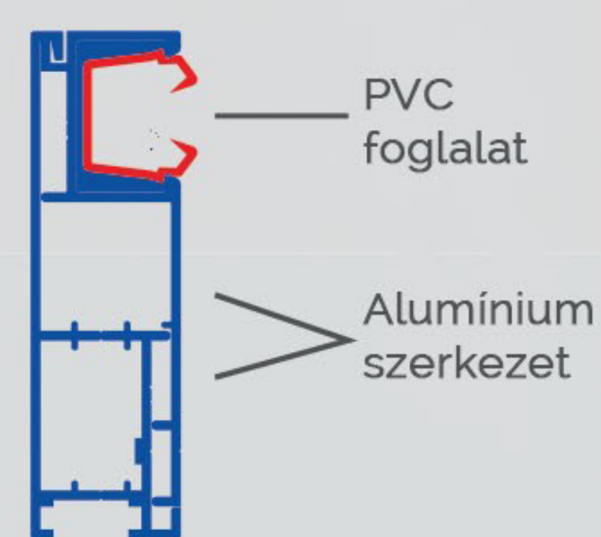
Alumínium vezetősin
